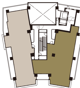
26階平面図
